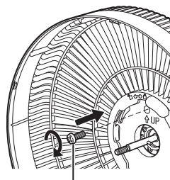
後ガード固定ネジ
